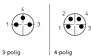
Pinbelegung für M8-Stecker, A-kodiert, Frontansicht
